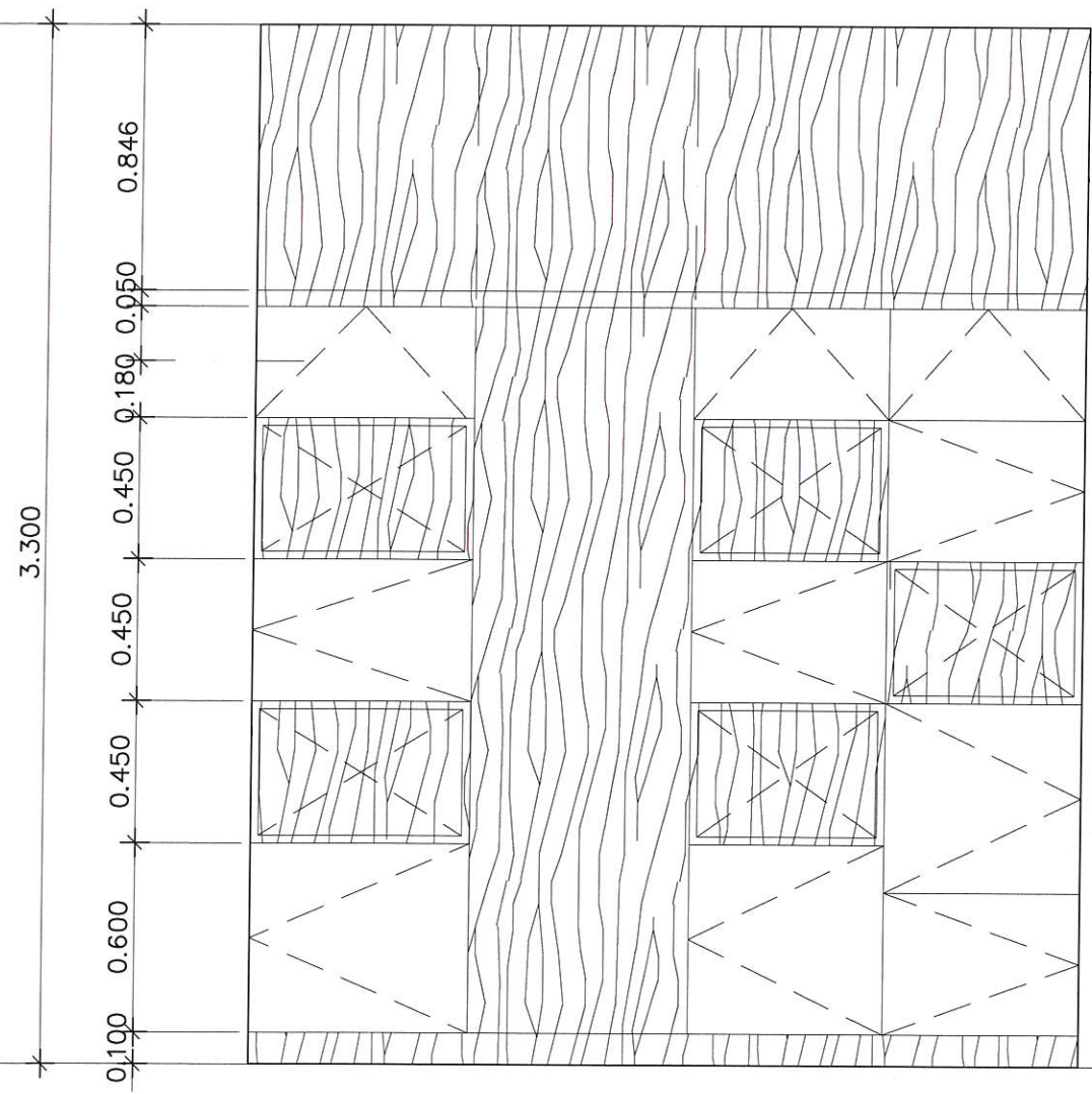
รูปด้าน SCALE 1:25
