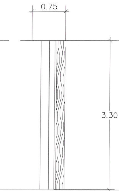
รูปตัด SCALE 1:50
