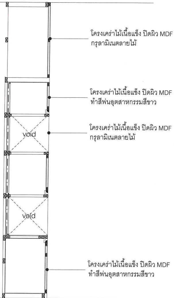
รูปตัด SCALE 1:25
