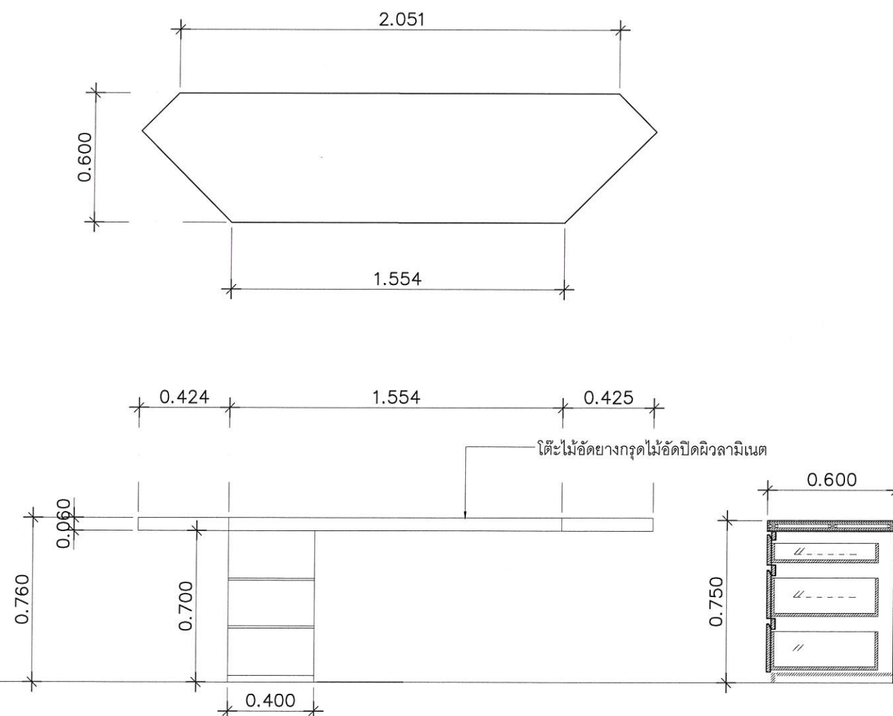
รูปด้าน SCALE 1:25
