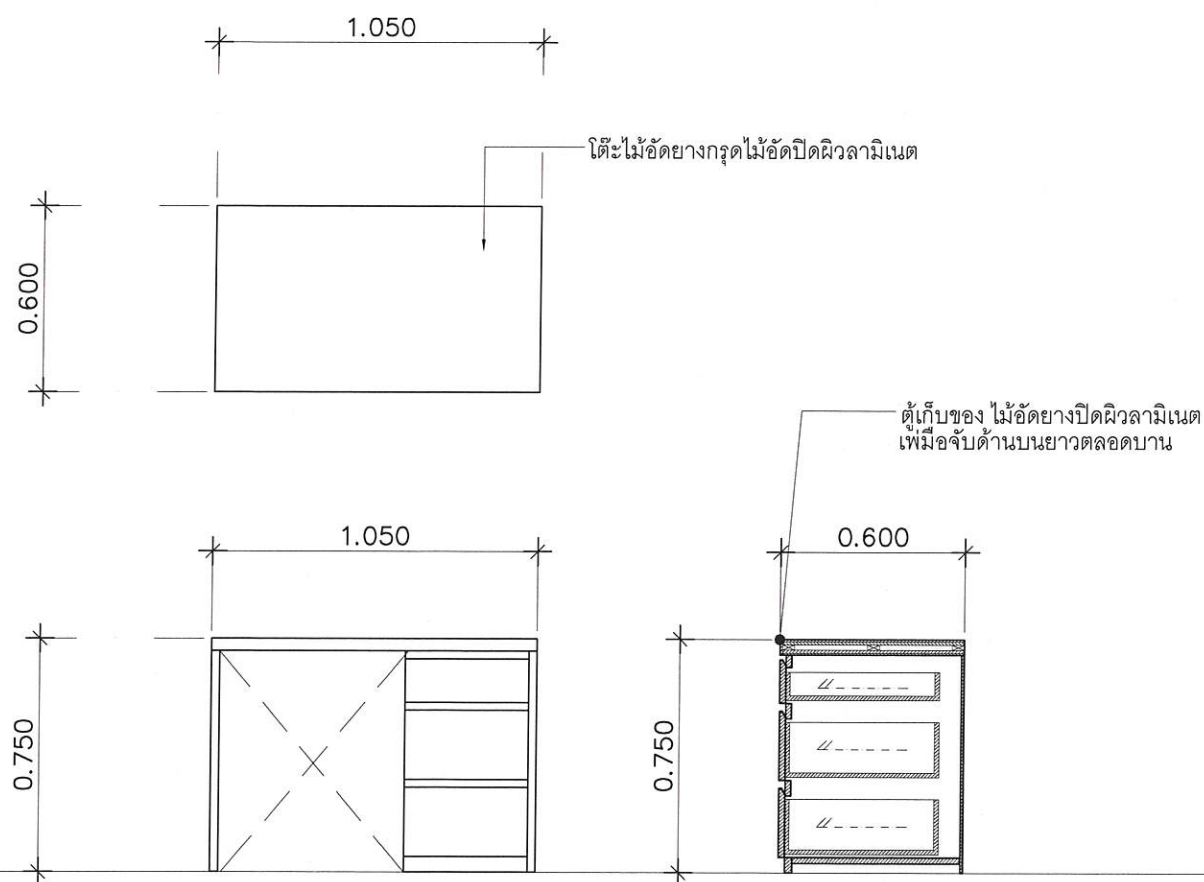
รูปด้าน SCALE 1:25
